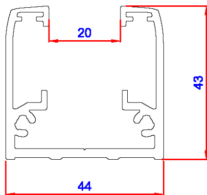
Perfil MARCO INFERIOR H43
