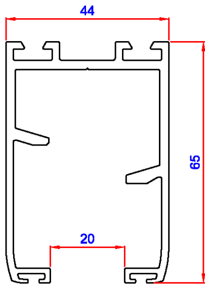
Perfil MARCO SUPERIOR
