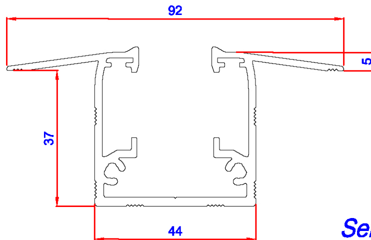
Perfil MARCO INFERIOR EMBUTIDO H43
