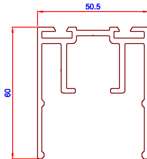
Perfil EXPANSOR
