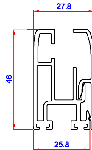
Perfil HOJA - JUNQUILLO
