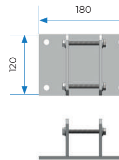
Fijación a suelo atornillado 180x120mm
