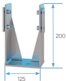
Supporto regolabile
