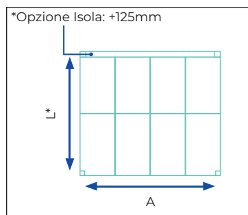
Struttura Seesky LUZ in configurazione isola
