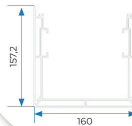
A1 PILASTRO "U" REGISTRABILE
