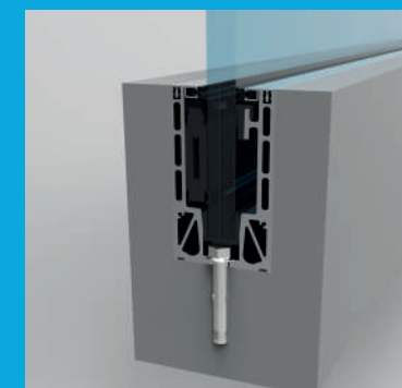
Opción empotrado Opção incrustado
