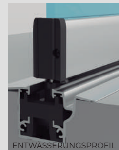
ENTWÄSSERUNGSPROFIL
