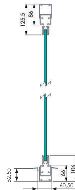
Oberer/unterer Rahmen mit eingelassenen Ausgleichprofil und Kondenswasser-rinne Einstellung: oben. +/-8 unten. +5/-25
