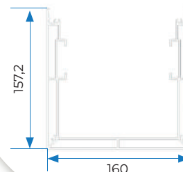
A1 | PILASTRO "U" REGISTRABILE
