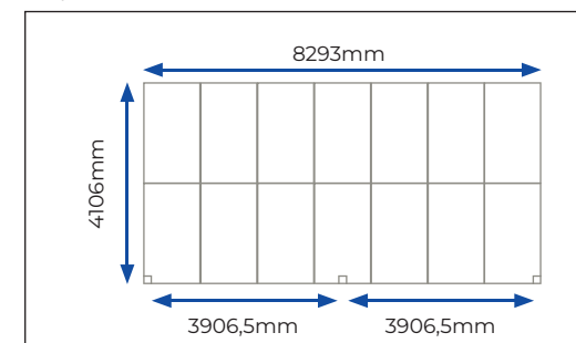
Struttura e-Orbita LUZ in configurazione a capanno
