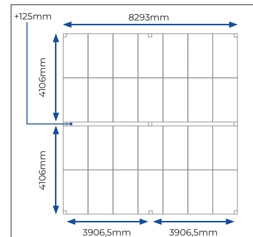
Struttura e-Orbita LUZ in configurazione a capanno
