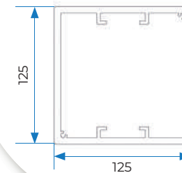
B1 | PROFILO PILASTRO CHIUSO
