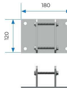
Fissaggio a pavimento con viti 180x120mm
