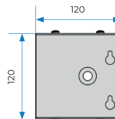
Unione a parete 120x120mm
