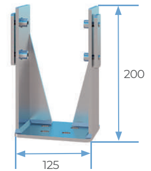
Regulierbare Stütze
