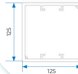
A2 | PERFIL PILAR CERRADO
