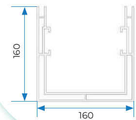
A2 | PERFIL PILAR U
