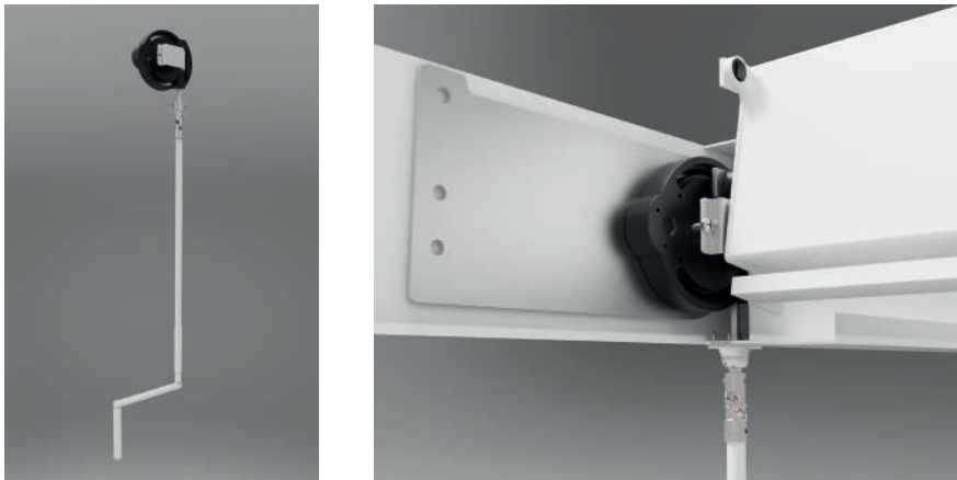
Kit manivela + cardán: Testado a +4000 ciclos de apertura/cierre
