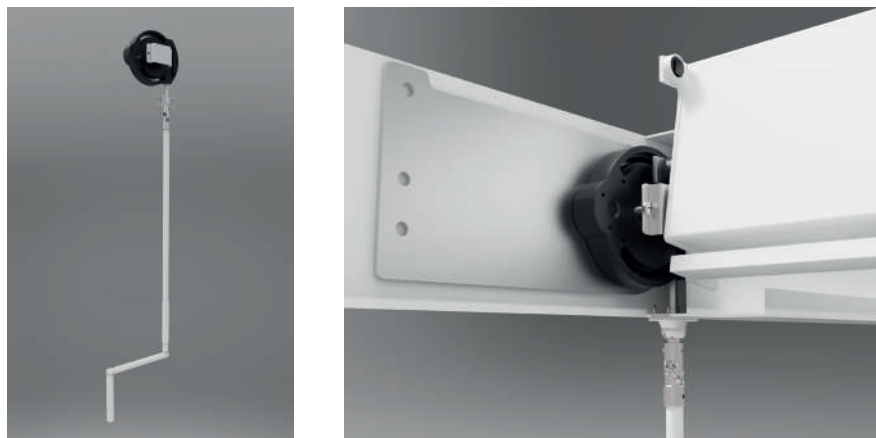
Kit manivela + cardã: Testado a mais de 4000 ciclos de abertura/fecho
