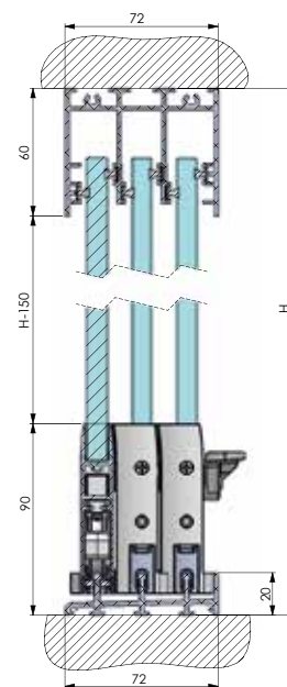
Sección sistema 3 carriles
